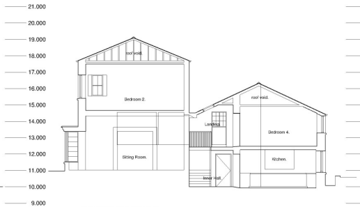
'AS EXISTING' SECTION B - B.
